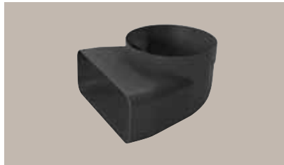
HZ9VDSI1 kolenová redukcia 90° na pripojenie plochého potrubia a kruhových prvkov potrubia s Ø 150 mm (samec)
