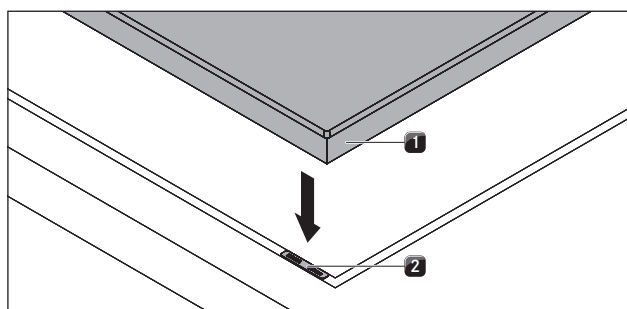
Obr. 5.15 Varná deska a podložky na nastavení výšky
