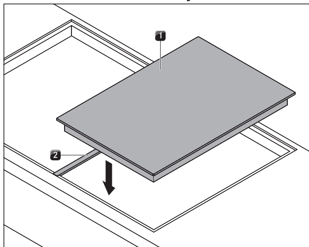
Obr. 5.14 Vložení montážní lišty a varné desky
