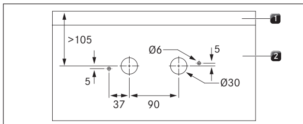
Obr. 5.9 Šablona otvorů
