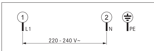
Obr. 5.17 Schéma zapojení 1-fázové
