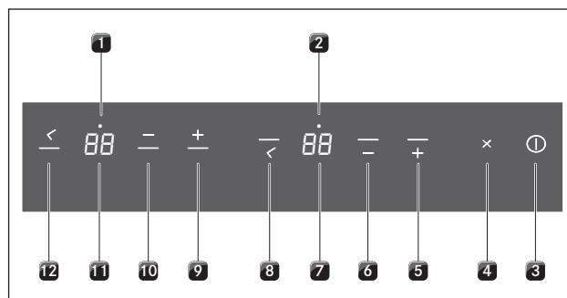
Obr. 4.2 Ovládací panel
