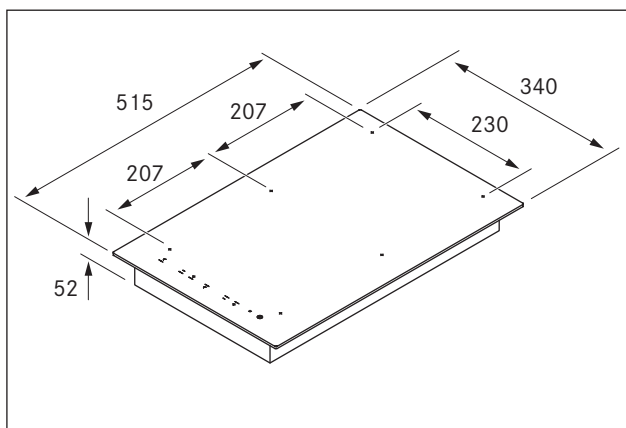
Obr. 3.1 Rozměry přístroje
