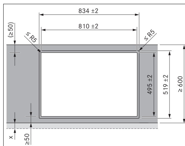
Obr. 6.7 Rozměry výřezu pro plošně zarovnanou montáž
