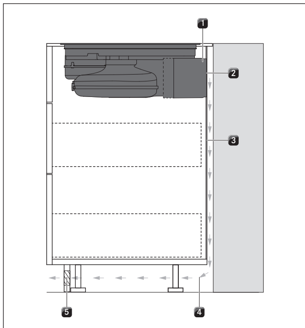
Obr. 6.25 Varianta montáže s průchozí zadní stěnou
