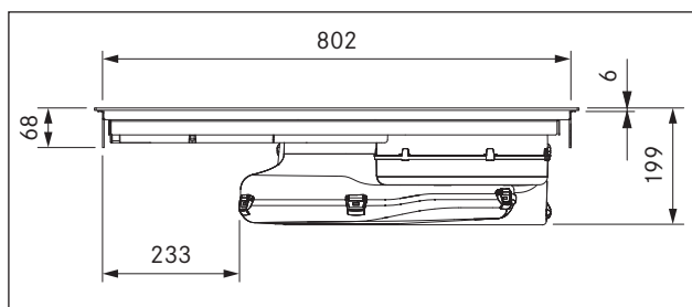
Obr. 3.5 Rozměry spotřebiče PUXU – pohled zepředu
