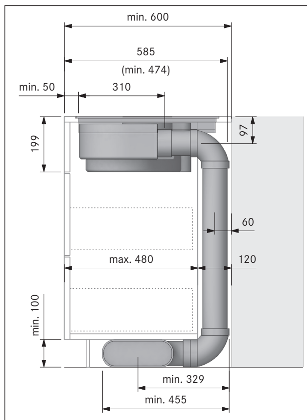
Obr. 6.15 Rozměry montáže při odtahu ven, hloubka pracovní desky 600 mm
