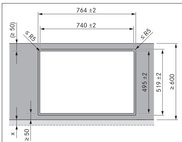
Obr. 6.11 Rozměry výřezu pro plošně zarovnanou montáž
