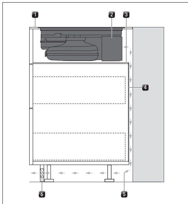
Obr. 6.26 Varianta montáže s vloženým dnem
