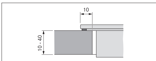
Obr. 6.14 Rozměry podkladu pro montáž na povrch
