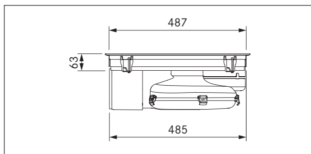
Obr. 3.13 Rozměry spotřebiče PURU – pohled z boku
