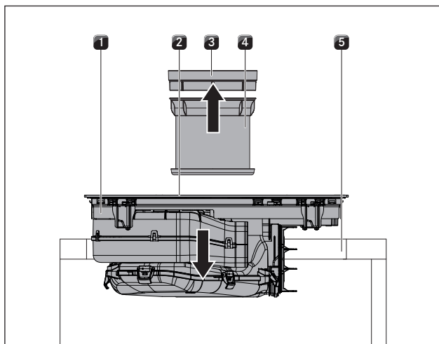
Obr. 6.19 Nasazení varné desky
