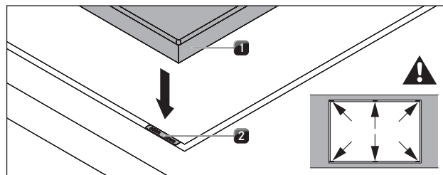
Obr. 6.20 Vložení podložky k nastavení výšky
