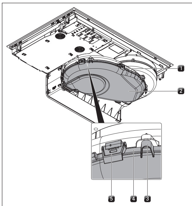
Obr. 8.4 Skříň ventilace
