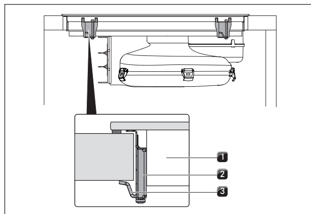
Obr. 6.22 Upevnění varné desky do středu
