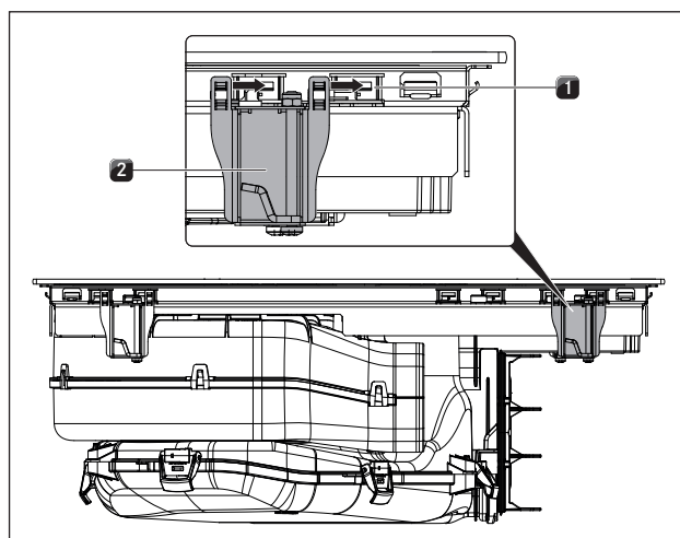
Obr. 6.33 Umístění montážních svorek
