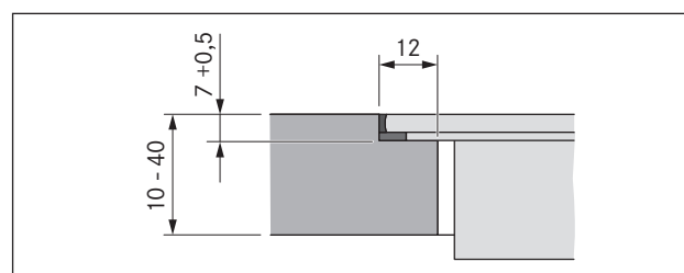
Obr. 6.8 Rozměr drážky pro plošně zarovnanou montáž
