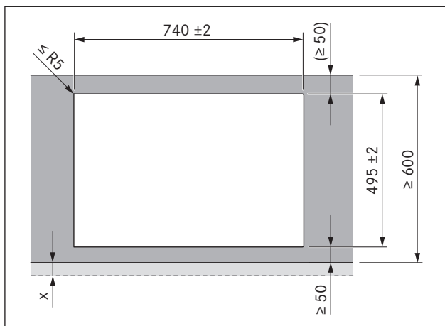
Obr. 6.13 Rozměry výřezu pro montáž na povrch
