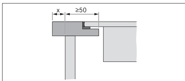
Obr. 6.6 Přesah pracovní desky
