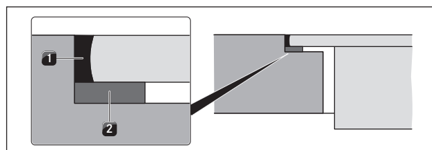
Obr. 6.17 Těsnicí páska při plošně zarovnané montáži
