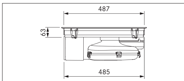
Obr. 3.6 Rozměry spotřebiče PUXU – pohled z boku
