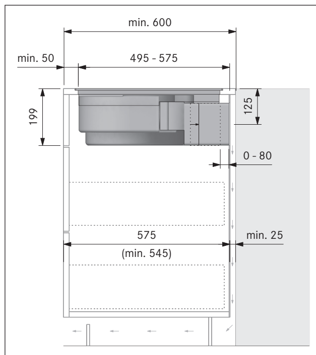
Obr. 6.27 Rozměry montáže u recirkulujícího vzduchu, varianta montáže A
