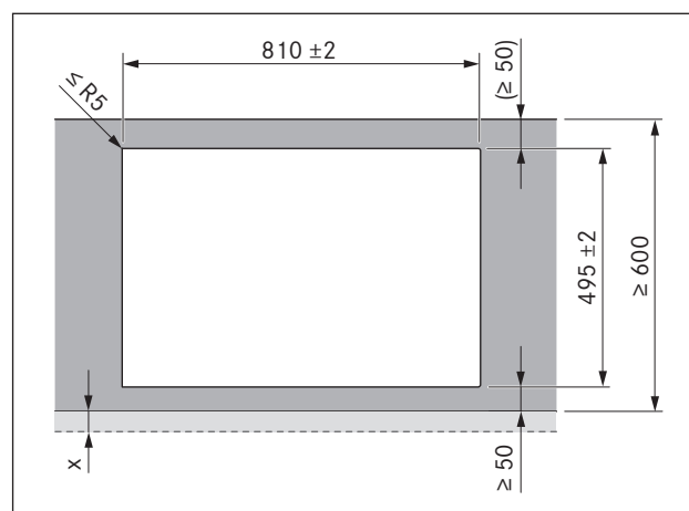
Obr. 6.9 Rozměry výřezu pro montáž na povrch
