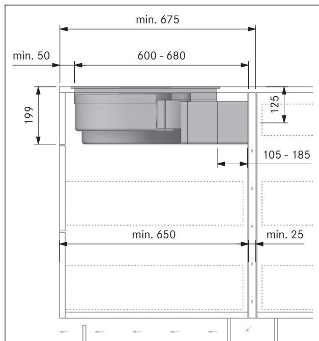
Obr. 6.34 Rozměry montáže u varianty montáže A, hloubka pracovní desky od 675 mm
