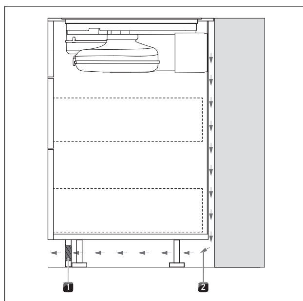
Obr. 6.24 Otvor na zpětné proudění vzduchu v oblasti soklu
