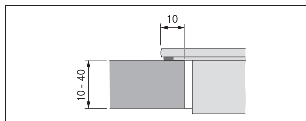
Obr. 6.10 Rozměry podkladu pro montáž na povrch
