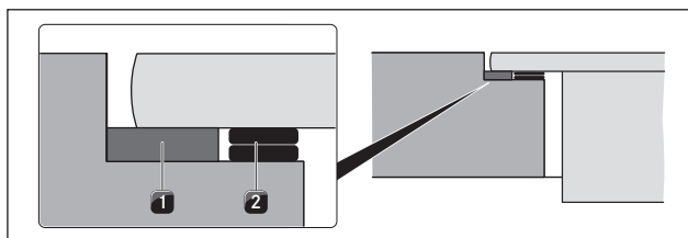
Obr. 6.38 Podložky k nastavení výšky
