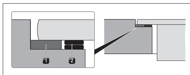
Obr. 6.21 Podložky k nastavení výšky
