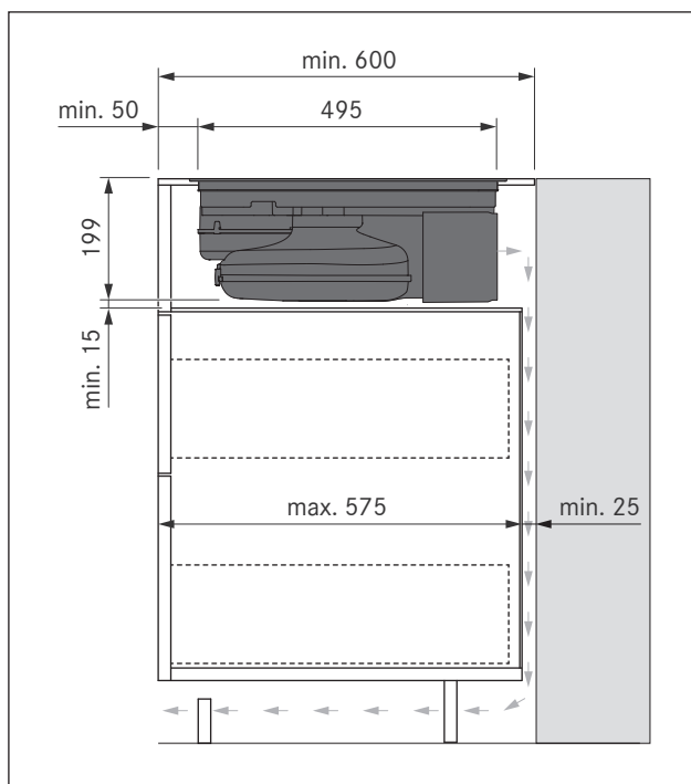
Obr. 6.30 Rozměry montáže u varianty montáže B, hloubka pracovní desky 600 mm
