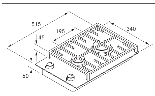
Obr. 3.1 Rozměry přístroje
