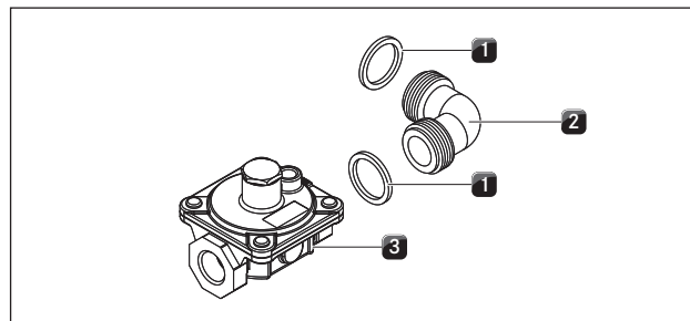
Obr. 6.1 Přípojka s regulátorem plynu (NG)
