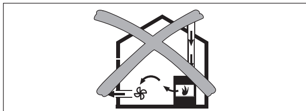
Obr. 6.19 Montáž odsávání – není přípustná
