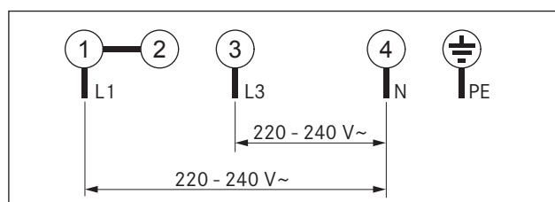
Obr. 6.37 Schéma zapojení 2-fázové přípojky
