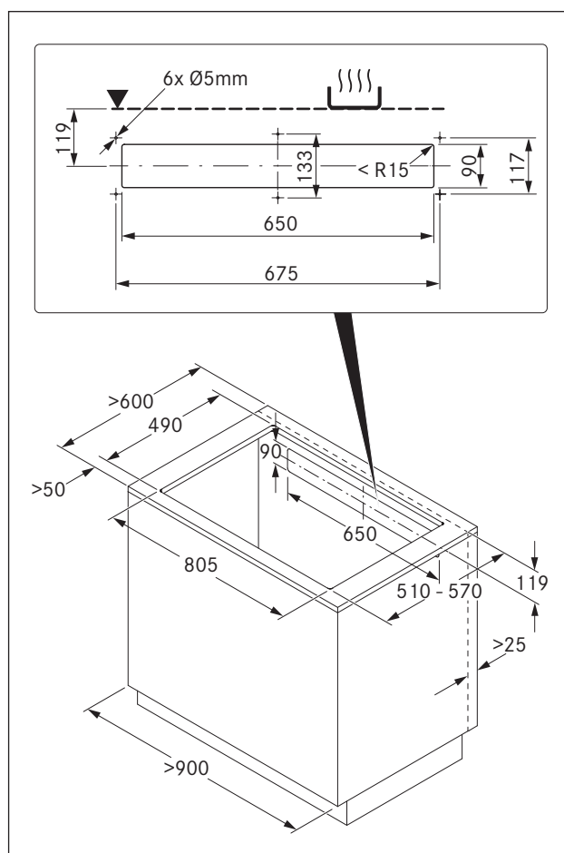
Obr. 6.10 Rozměry nábytku u provedení s recirkulací
