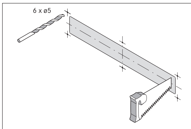
Obr. 6.12 Výřez a připojovací otvory
