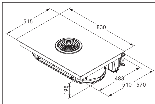
Obr. 6.9 Rozměry spotřebiče v provedení s recirkulací
