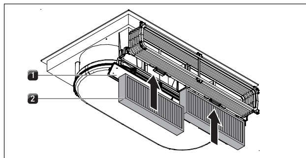
Obr. 6.17 Nasazení filtru s aktivním uhlím
