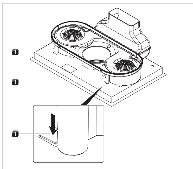
Obr. 6.26 Odjištění pojistky polohy
