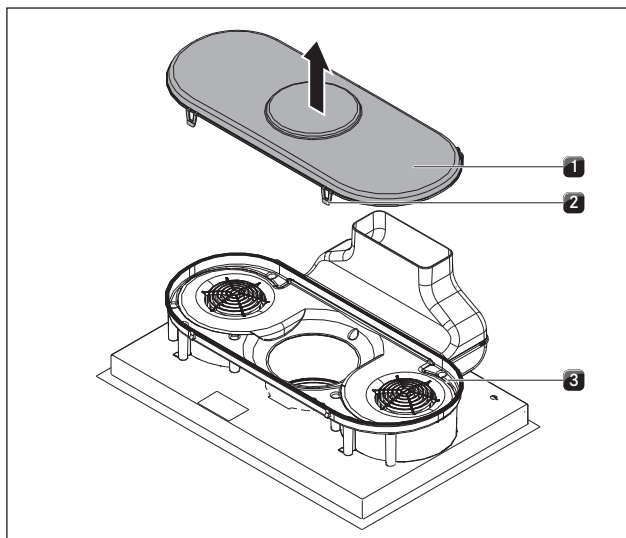
Obr. 6.25 Odejmутí dna skříně
