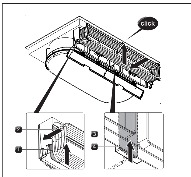
Obr. 6.16 Zavěšení rámu flex-kanálu
