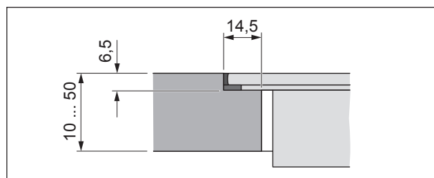
Obr. 6.3 Rozměr drážky pro plošně zarovnanou montáž
