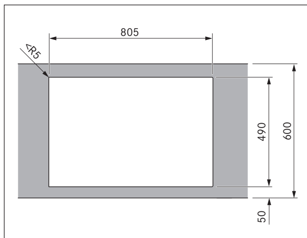
Obr. 6.4 Rozměry výřezu pro montáž na povrch
