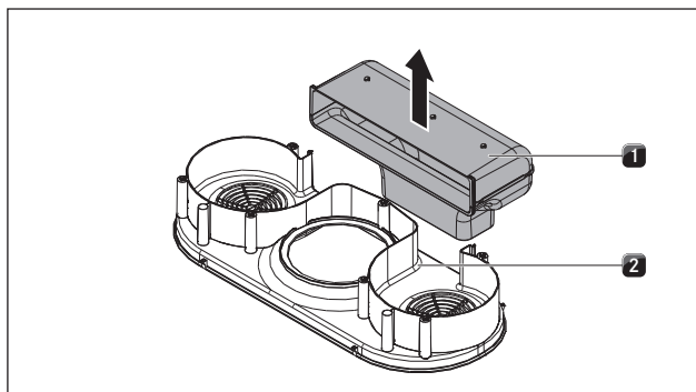
Obr. 6.29 Sejmutí odtahového kolene
