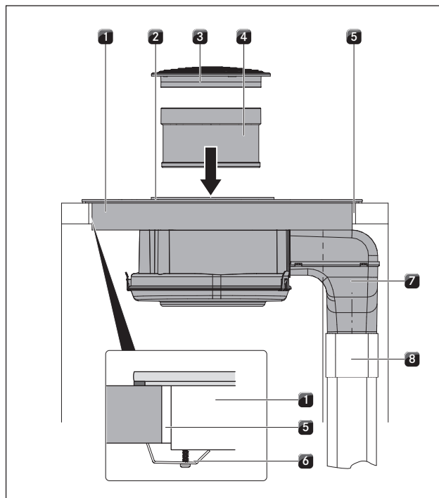
Obr. 6.35 Připojení odtahového kanálu
