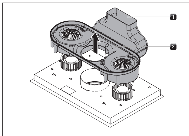
Obr. 6.28 Vyjmutí skříně vedení vzduchu
