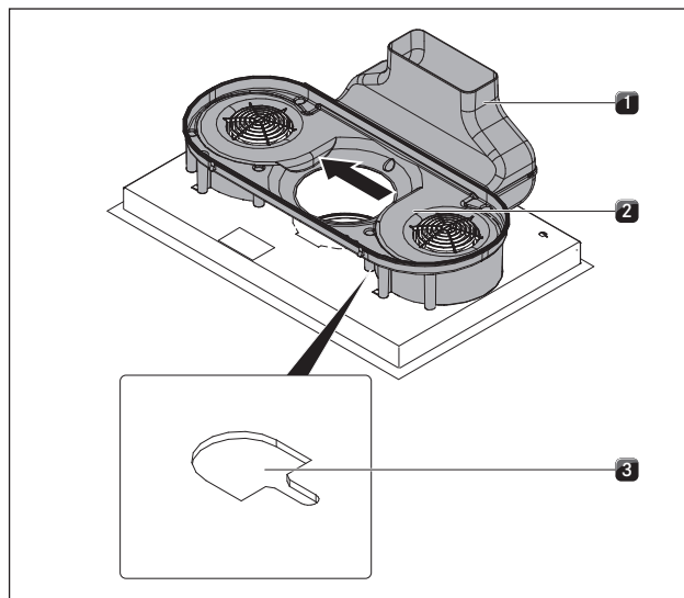
Obr. 6.27 Vysunutí skříně vedení vzduchu
