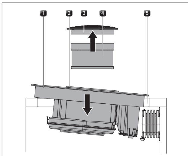
Obr. 6.14 Šikmé nasazení varné desky
