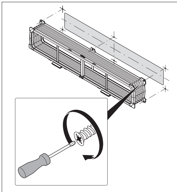
Obr. 6.13 Flex-kanál s 6 EURO šrouby 6,3 x 10 mm
