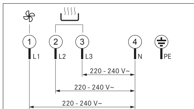
Obr. 6.36 Schéma zapojení 3-fázové přípojky
