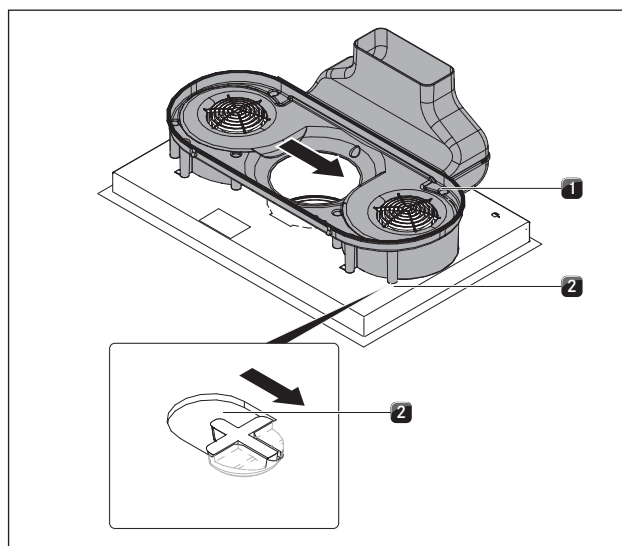
Obr. 6.32 Zcvaknutí jednotky vedení vzduchu
