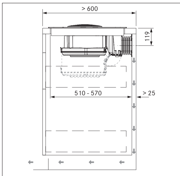
Obr. 6.11 Montážní rozměry pro provedení s recirkulací, hloubka pracovní desky 600 mm
