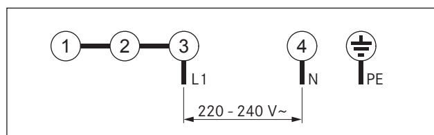
Obr. 6.38 Schéma zapojení 1-fázové přípojky
